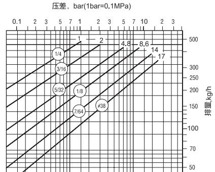
881 型排量图
