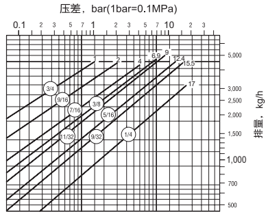
815 型排量图
