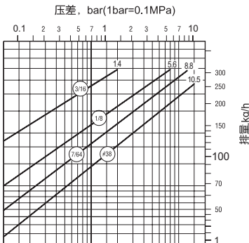
880 型排量图
