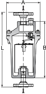
图2 200系列疏水阀
