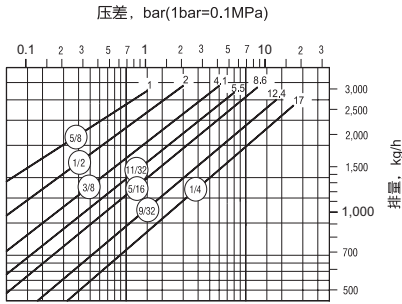
814 型排量图
