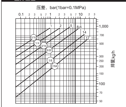
882 型排量图
