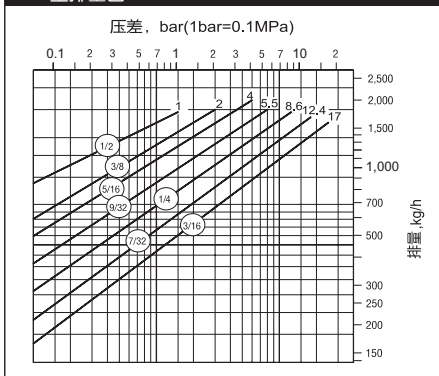
883 型排量图
