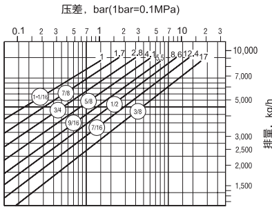
816 型排量图
